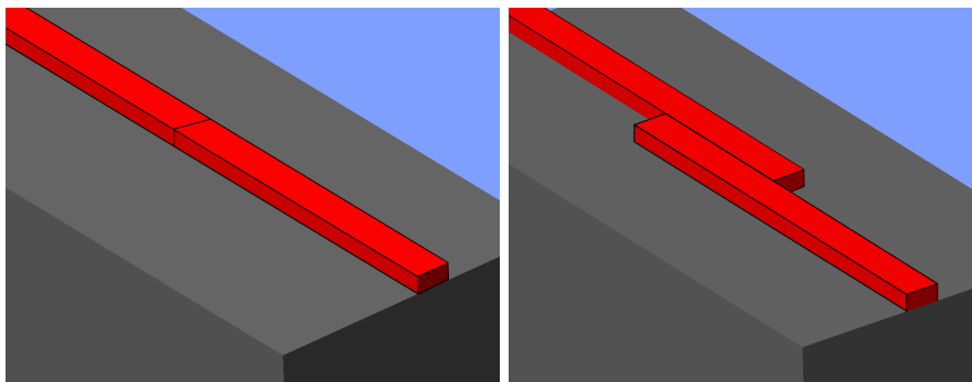
Rys. 1. Montaż kolejnych odcinków taśm Swell Sil
